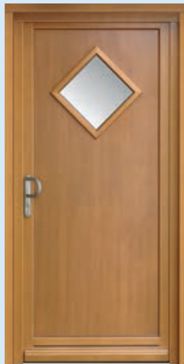
Holz Modell 30128 (PG23/31) Variante: Classic Glas: Klar plan Griff: HA7000 Wechselgarnitur mit Stoßgriff und schmalen Langschild Titan
